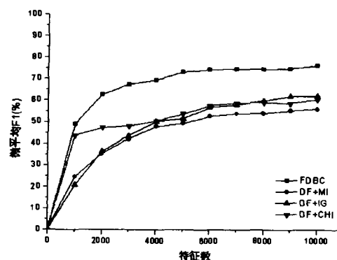
图2 四种方法微平均 F1 值的比较
