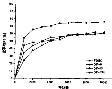
图1 四种方法宏平均 F1 值的比较
